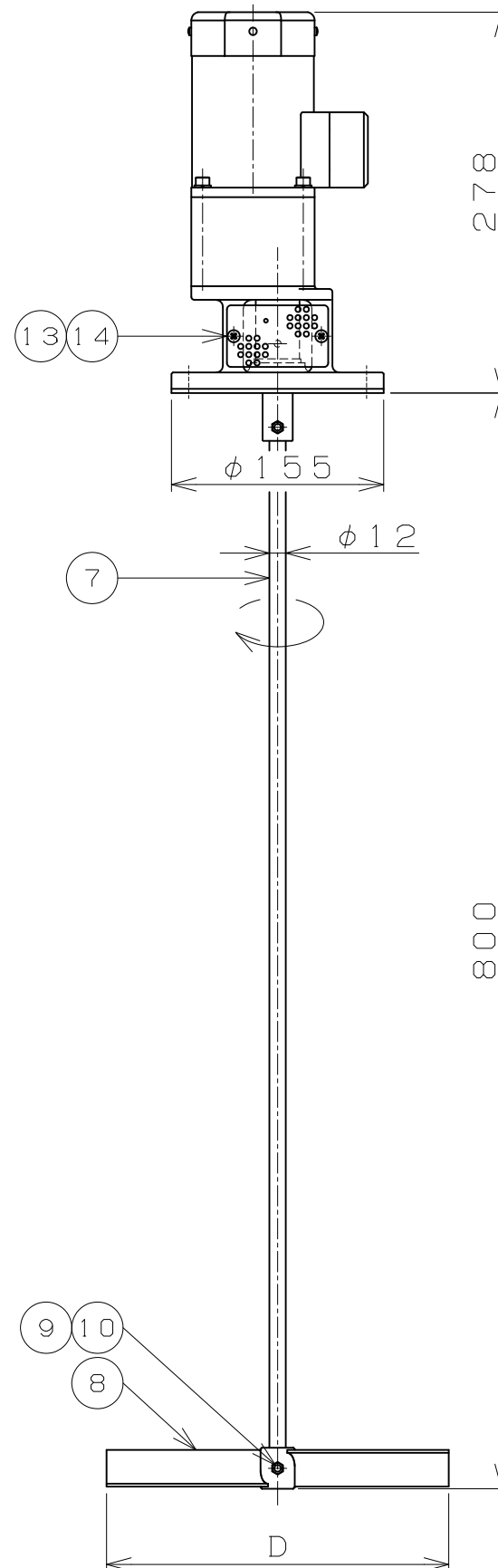
全体図 (S=1:5)
